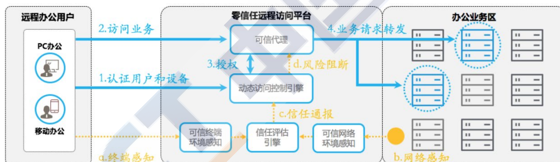
图3 基于零信任架构的远程办公安全参考架构
