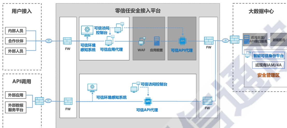
图 5 数据中心安全接入区案例示意图
