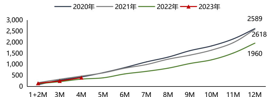
图19：2022年风电累计建设投资完成额月度变化情况（亿元）
