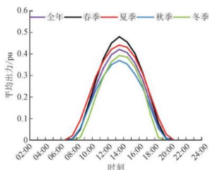
图8：光伏日平均出力曲线图
