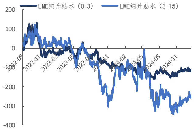
图表11: 铜期限结构(美元/吨)
