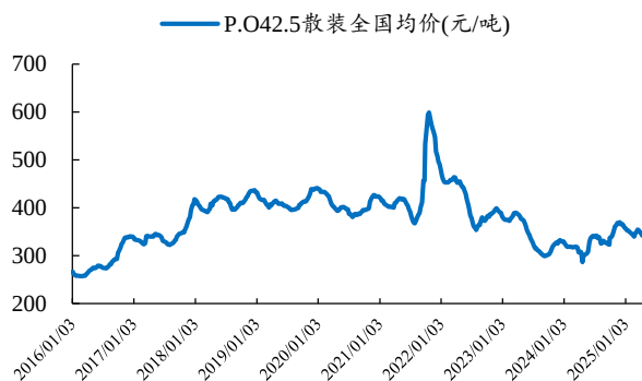
图8：本周全国 P.O42.5 水泥价格环比下跌 1.82%
