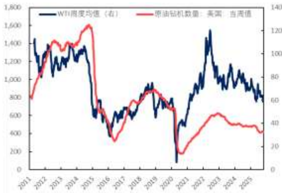
图 18：美国原油钻机数和油价走势（台，美元/桶）
