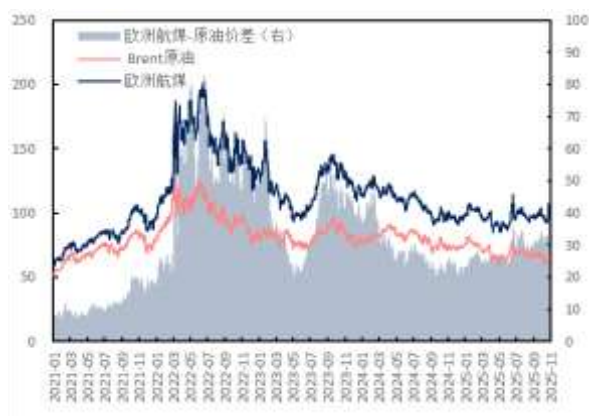
图 53: 原油、欧洲航煤价格及价差 (美元/桶, 美元/桶)
