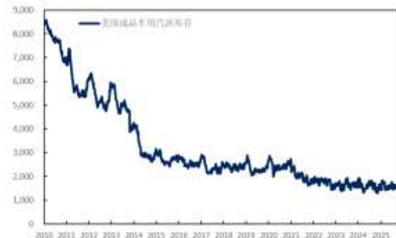
图 72: 美国成品车用汽油库存 (万桶)
