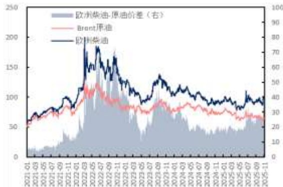
图 51：原油、欧洲柴油价格及价差（美元/桶，美元/桶）
