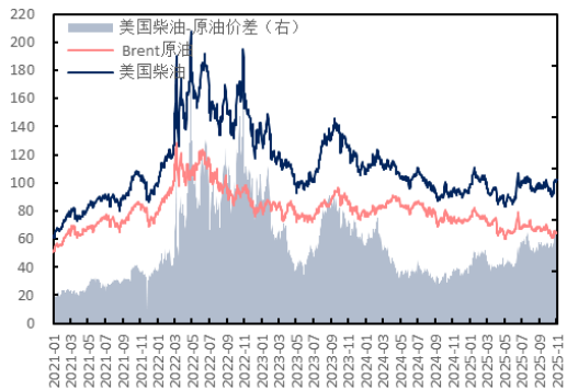
图 48：原油、美国柴油价格及价差（美元/桶，美元/桶）
