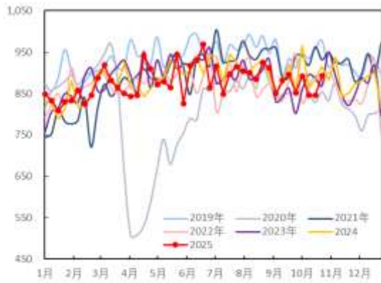
图 60：美国成品车用汽油消费量（万桶/天）
