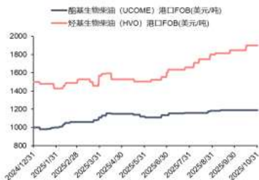
图 82：生物柴油港口 FOB 价格（美元/吨）
