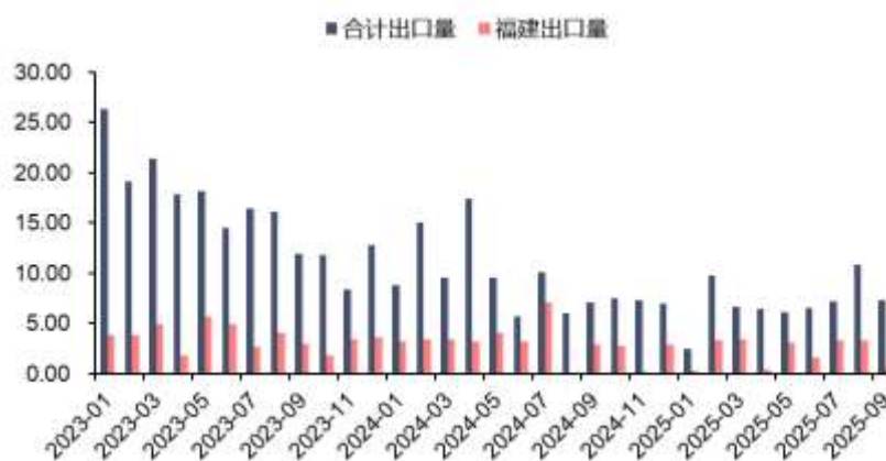
图 91: 酯基生物柴油月度出口量 (万吨)
