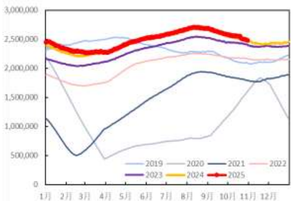
图 63：美国旅客机场安检数（人次）
