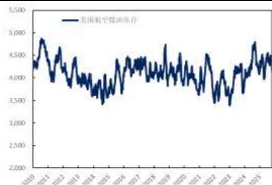
图 76: 美国航空煤油库存 (万桶)
