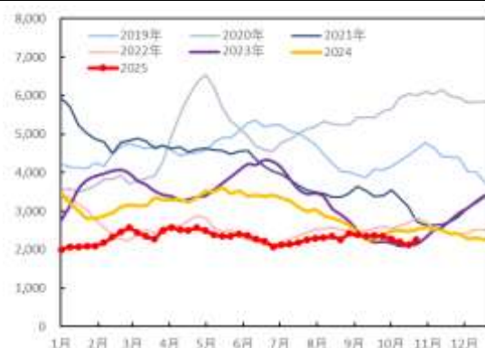
图 37: 美国库欣地区原油库存 (万桶)
