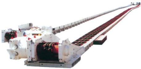
刮板输送机
