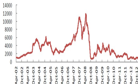
图 1：2002~2012 年 BDI 走势
