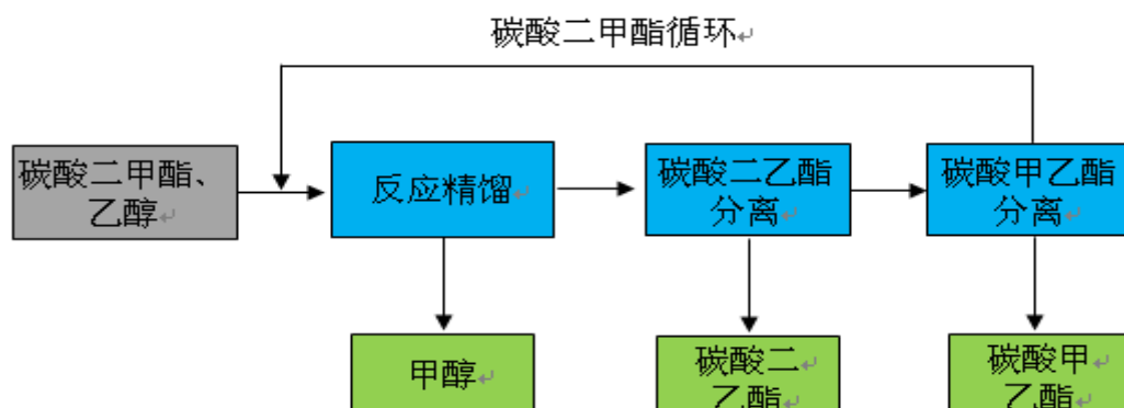
6、碳酸甲乙酯装置生产工艺流程图
