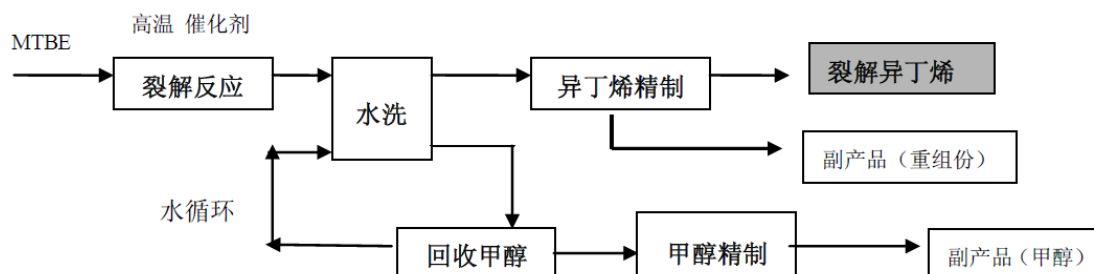
齐翔腾达的异丁烯生产工艺流程图
