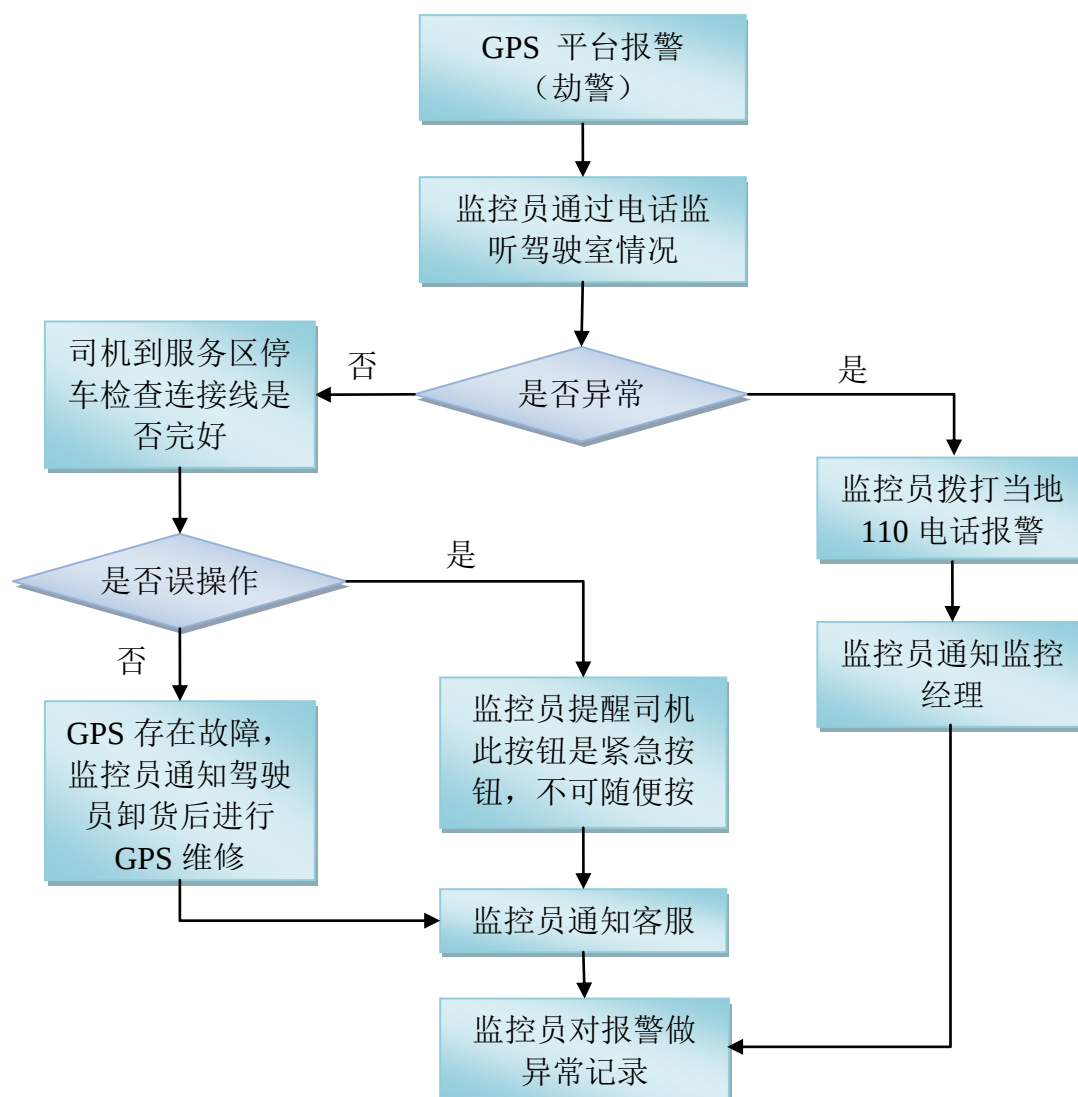
劫警报警处理流程图：
