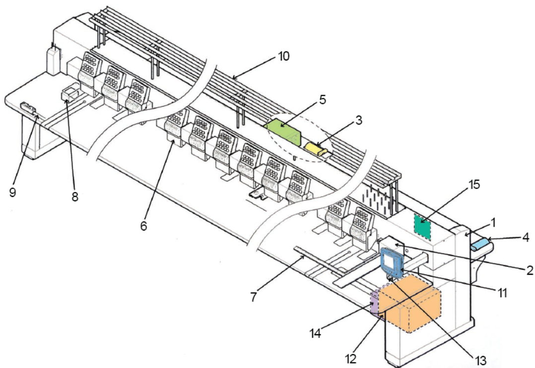
刺绣机电控系统结构示意图
