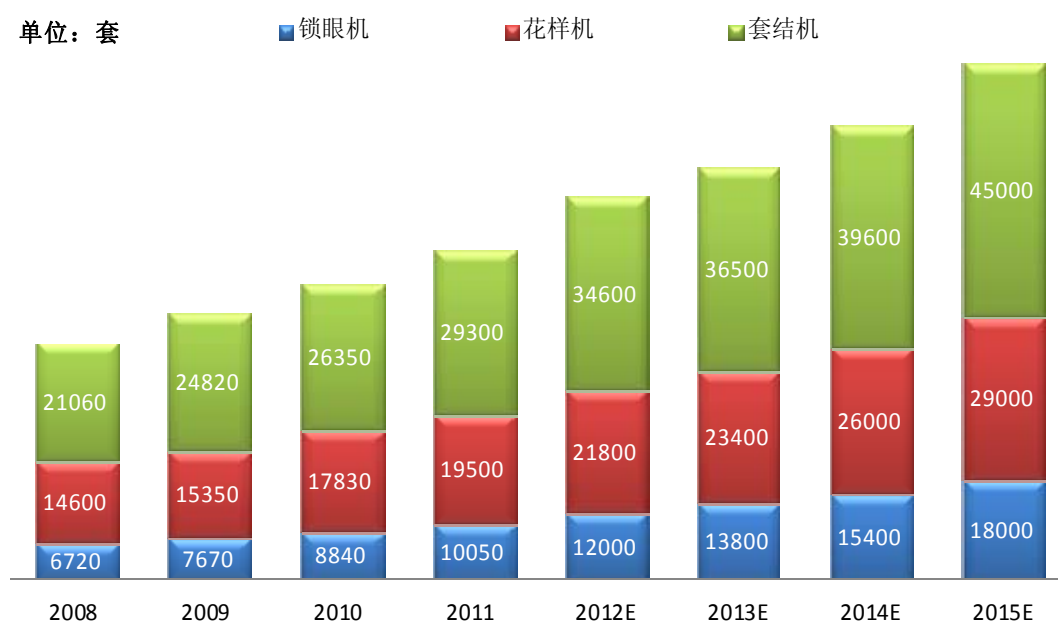
工缝机电控系统国内需求和预测
