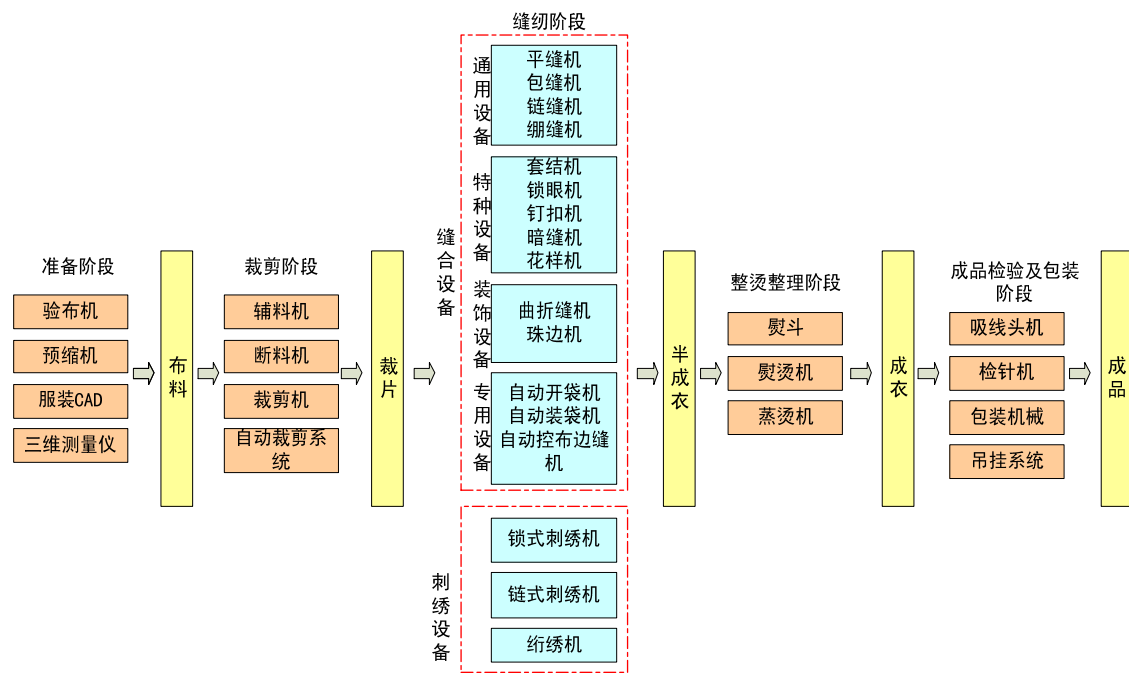
工业化服装生产中主要缝制机械设备功用示意图
