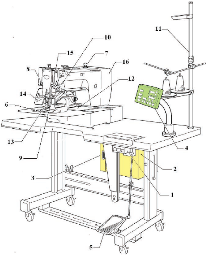
特种工业缝纫机电控系统结构示意图
