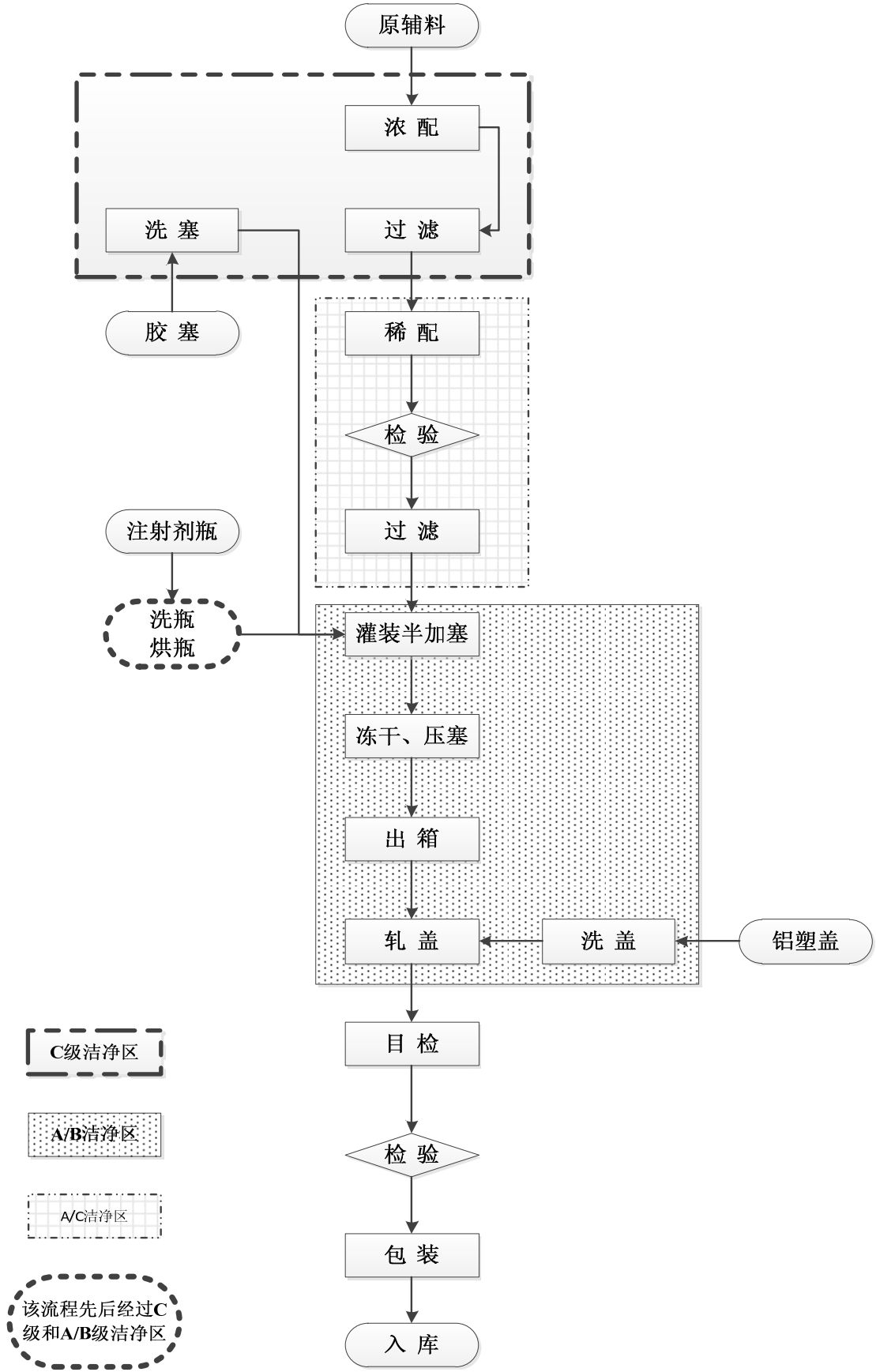
(2) 冻干粉注射液工艺流程图
