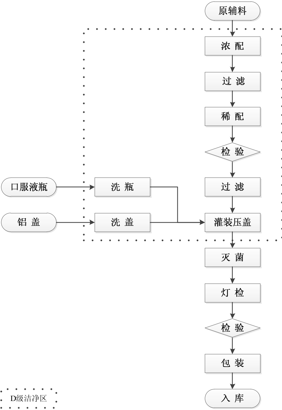
(3) 口服液工艺流程图
