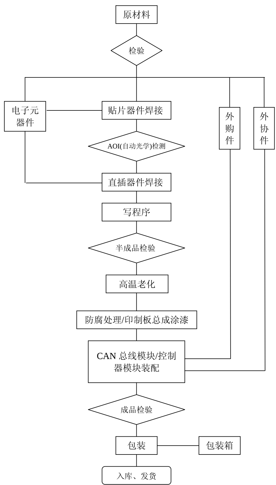
CAN 总线控制系统、控制器工艺流程图
