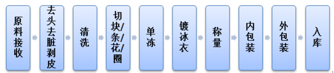
(5) 章鱼产品加工流程图
