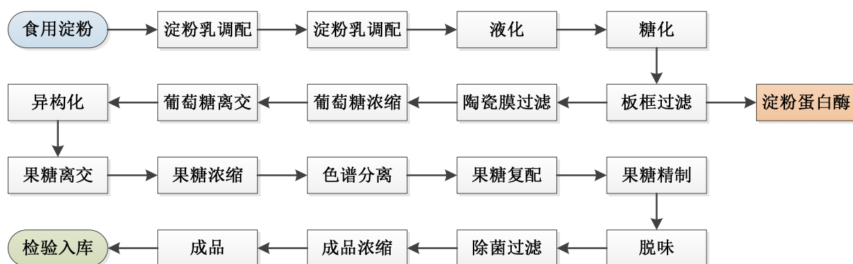
淀粉糖生产工艺流程图
