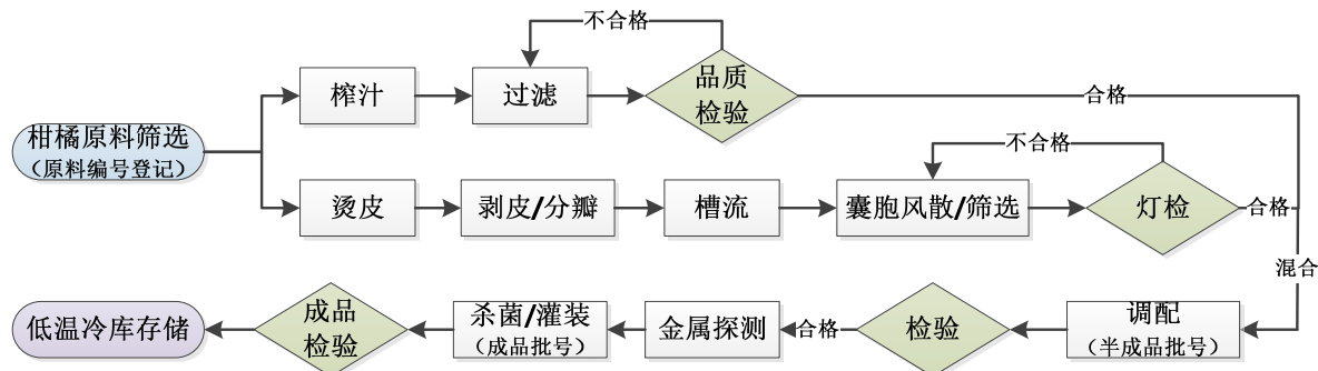
果汁囊胞生产工艺流程图
