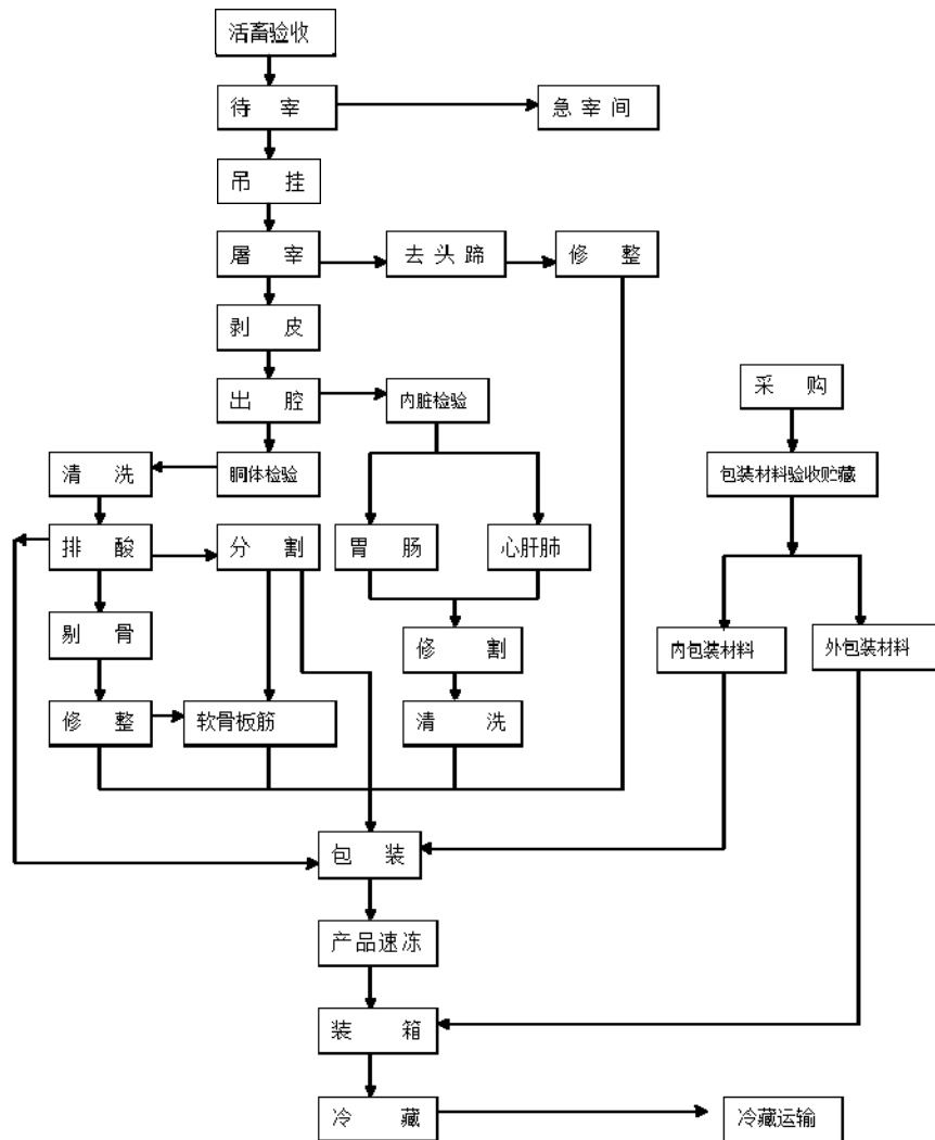
屠宰加工生产工艺流程图
