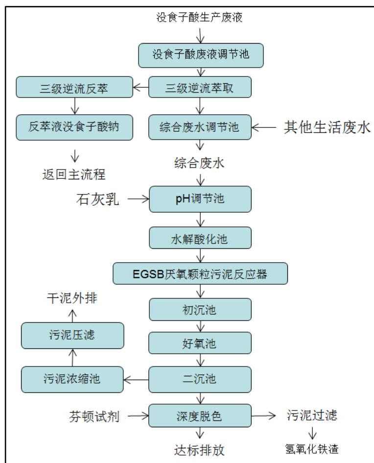
废液综合利用关键流程示意图
