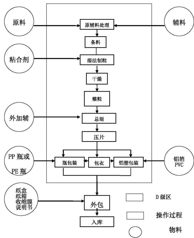
片剂工艺流程图
