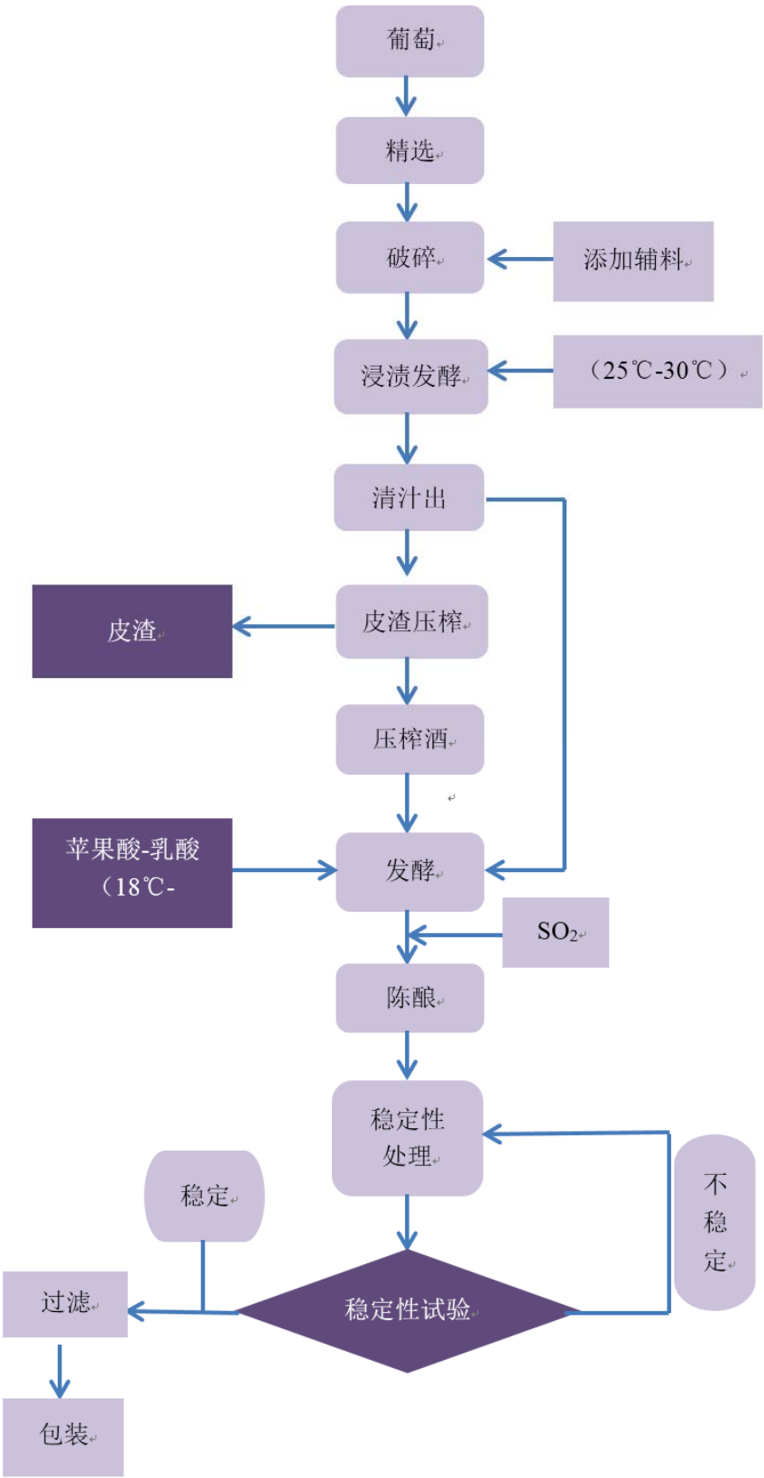
干红生产流程图
