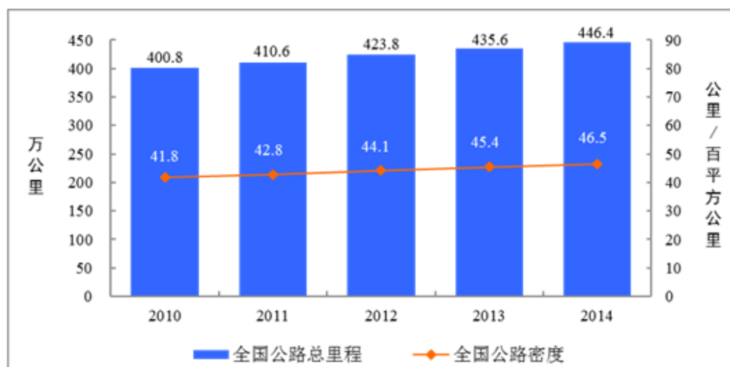
图 2 2010—2014 年全国公路总里程及公路密度
