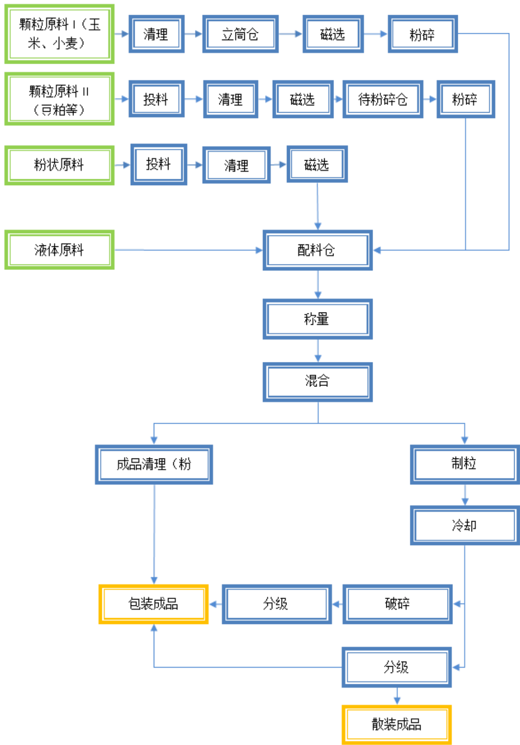
饲料生产加工流程图
