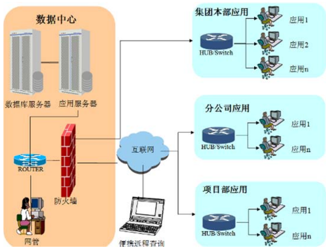
美芝股份信息技术平台网络拓扑图
