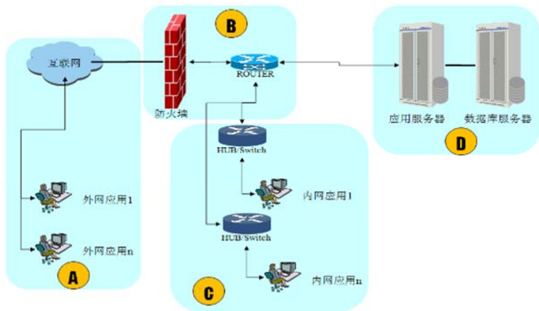
美芝股份信息技术平台网络拓扑图
