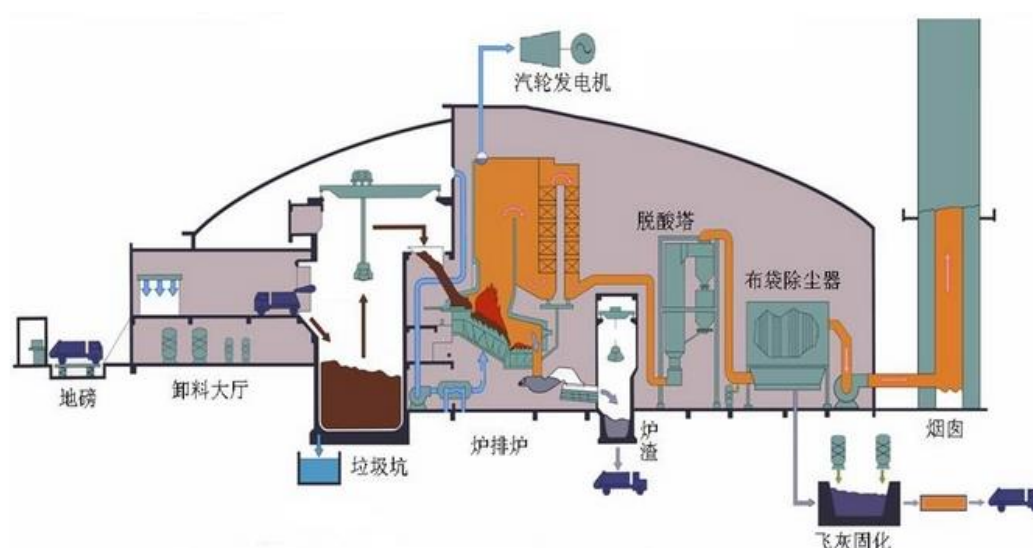
图 3-8 生活垃圾焚烧处理工艺流程（炉排炉）
