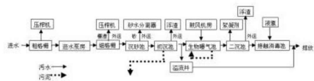
图 3-3 公司污水处理技术工艺流程图
