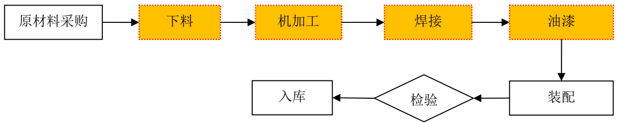
(7) 属具生产工艺流程
