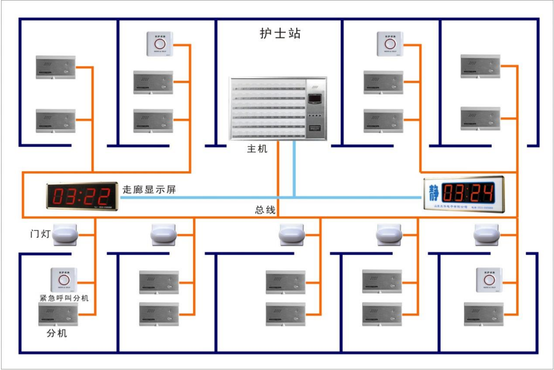
YH 系列智能护理通讯系统联网示意图
