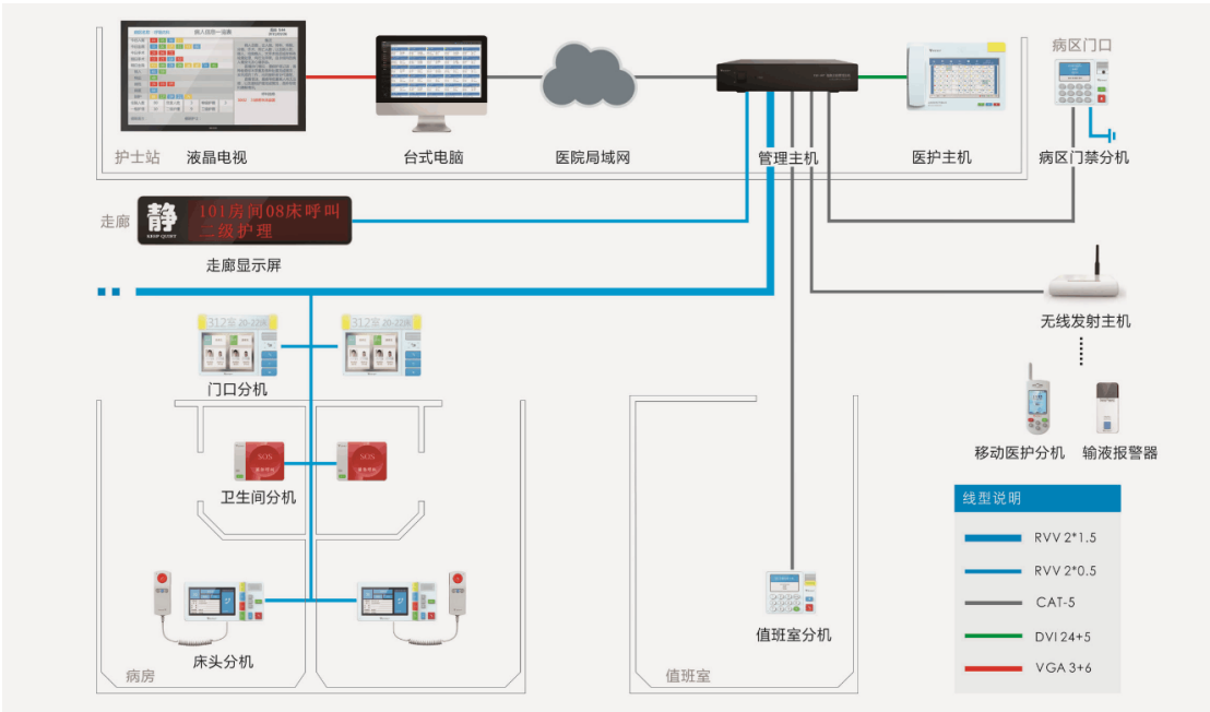
YH-997 系列信息化医护管理通信系统联网示意图
