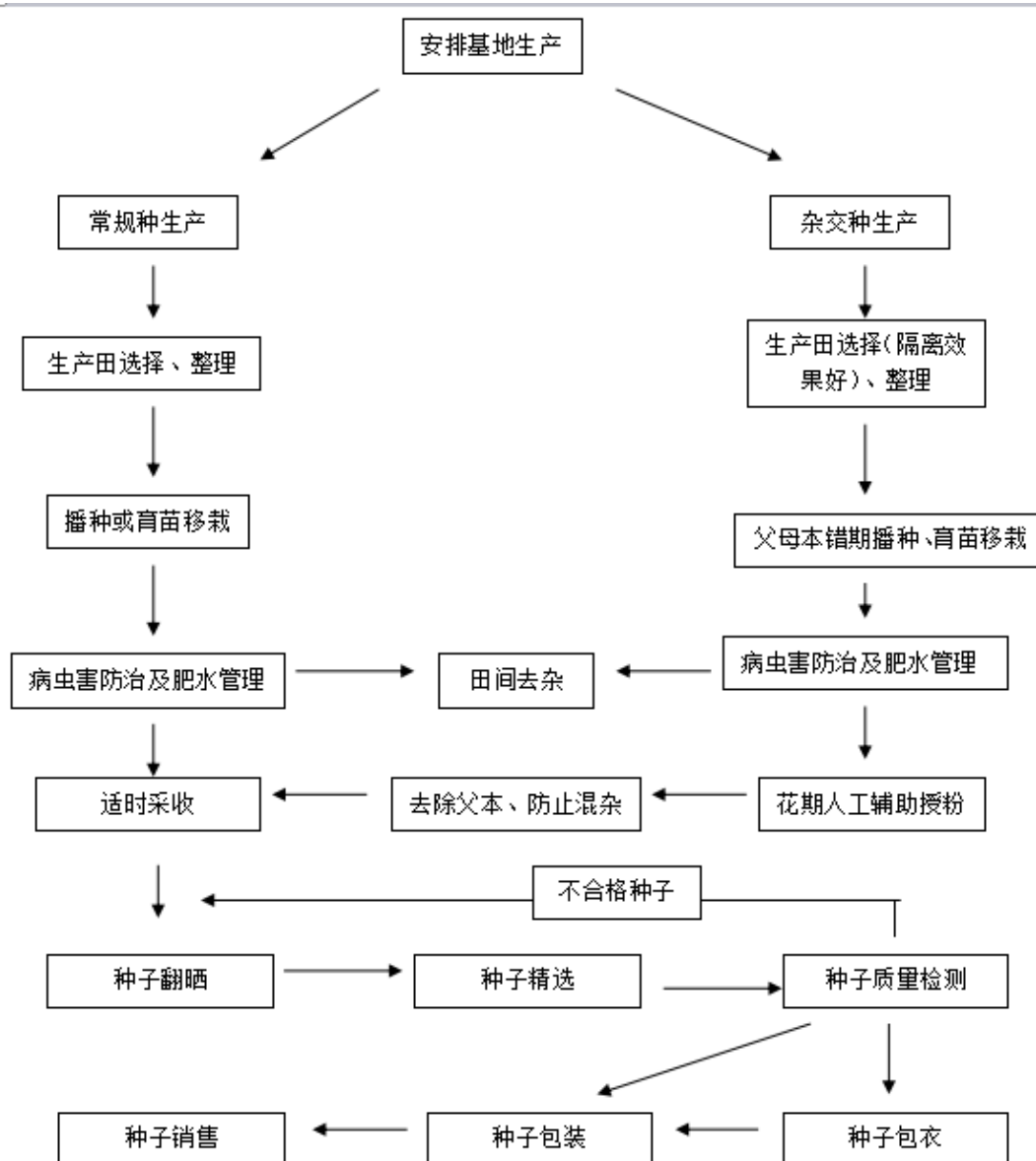
生产流程图：
