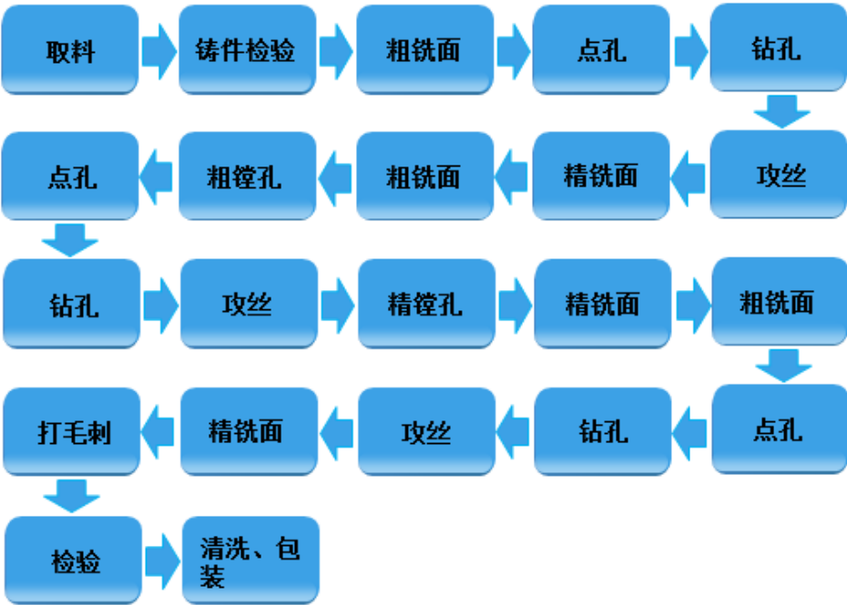
塑料机械铸件精加工工序流程图
