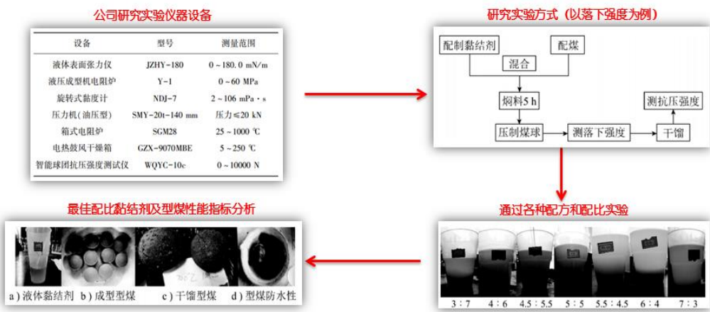
环保洁净型煤研究实验方式示意图
