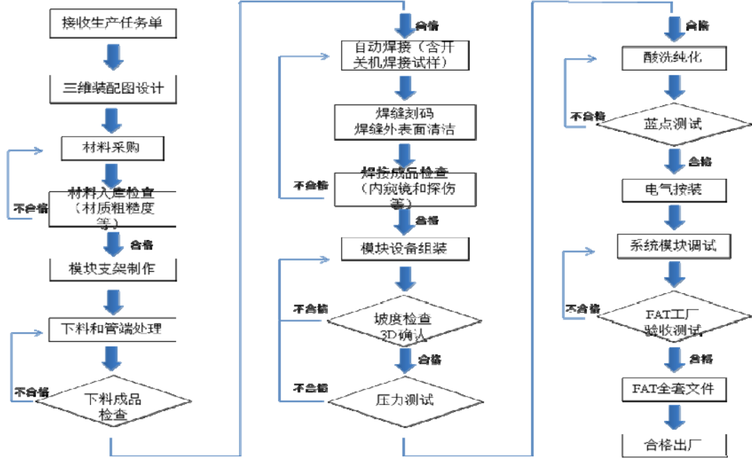
(3) 高纯工艺系统的现场作业流程如下表所示：
