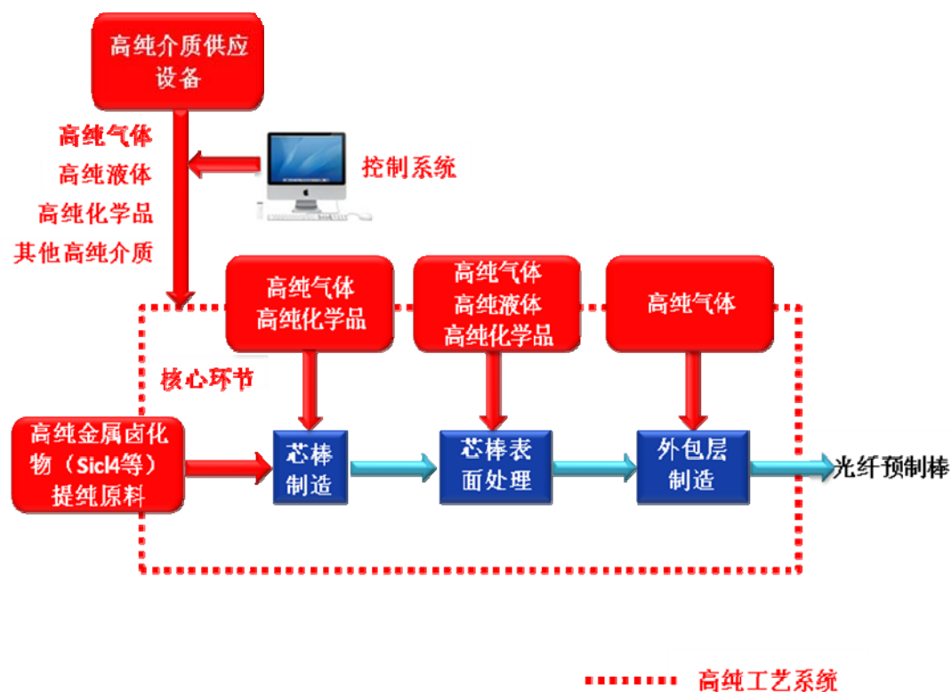
光纤预制棒核心工艺流程
