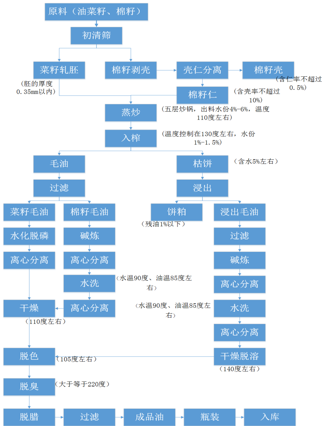
(2) 四级菜籽油生产流程（预榨、浸出法）
