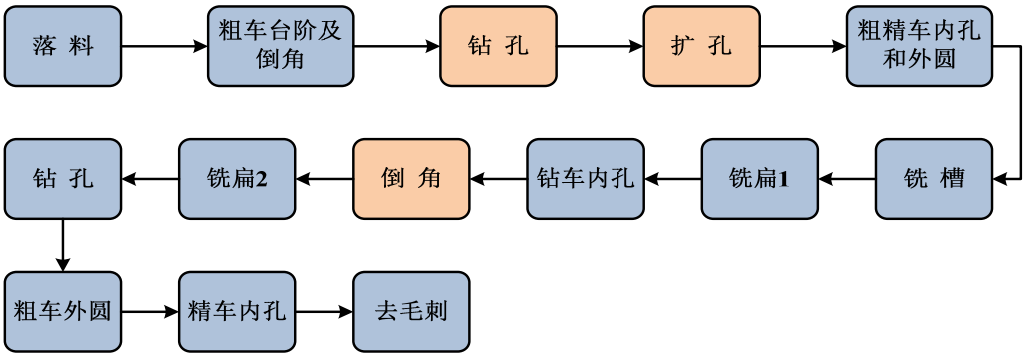
活塞类产品生产工艺流程改进图
