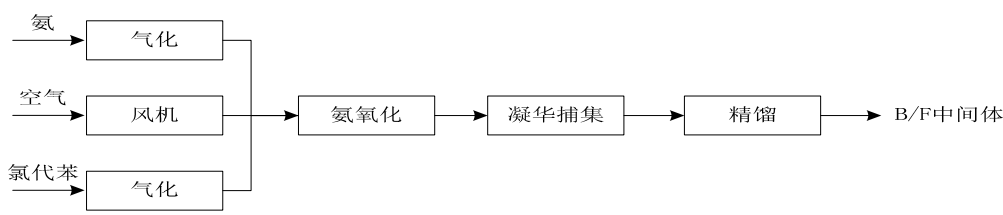
中间体 B/F 腈工艺流程图
