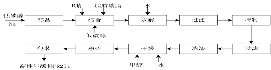
高性能颜料 PR254 工艺流程图
