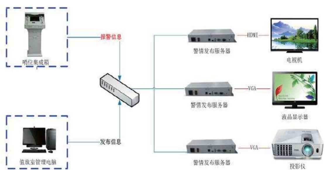
图 2.8 警情发布报警系统连接图
