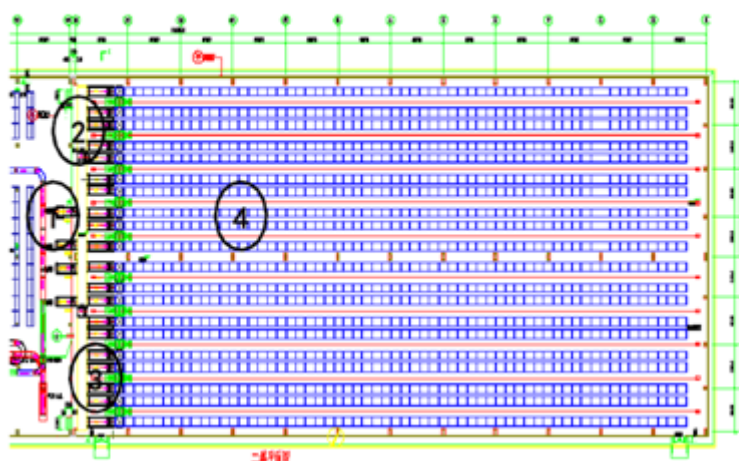
立库二楼的平面布置示意图
