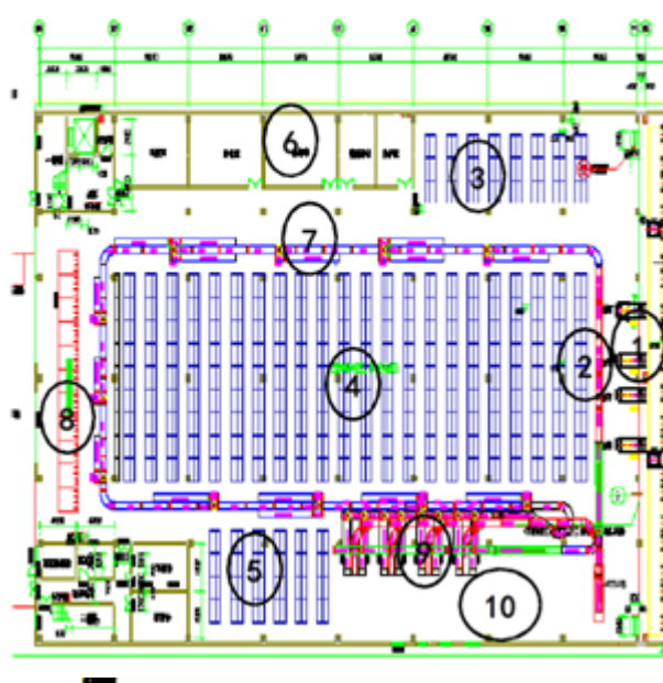
立库一楼的平面布置示意图
