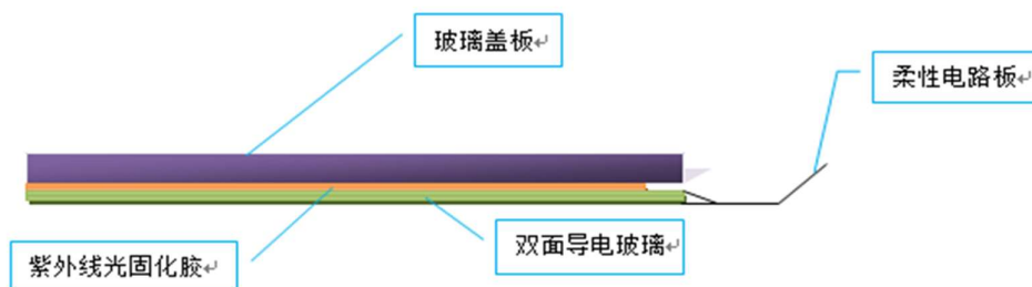
G+G 结构示意图
