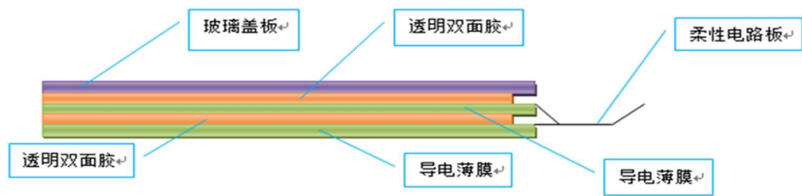
G+F+F 结构示意图
