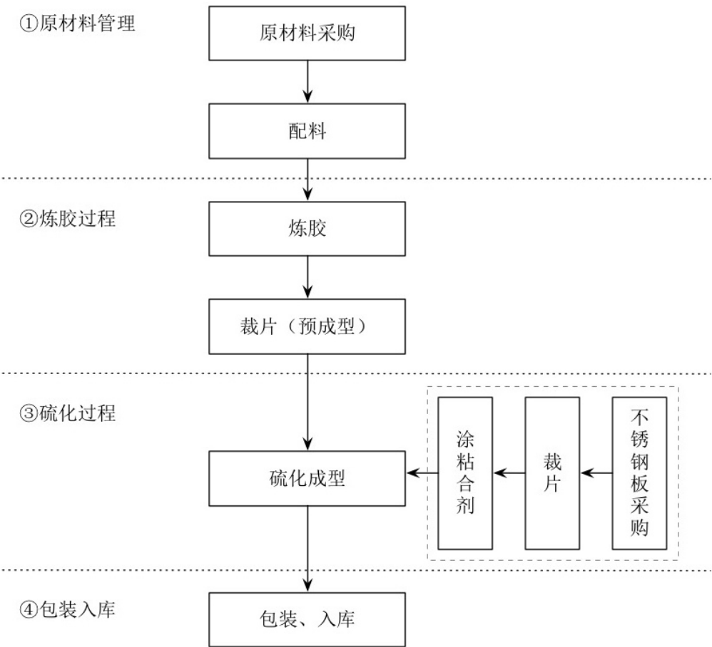
(3) 橡胶件生产工艺流程图
