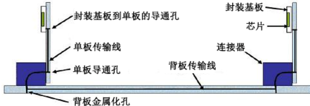
背板与单板组装截面图
