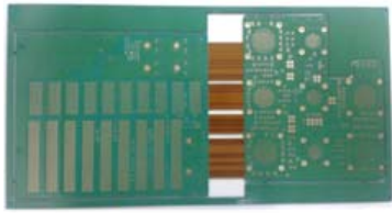
高多层Air-gap结构刚挠板
