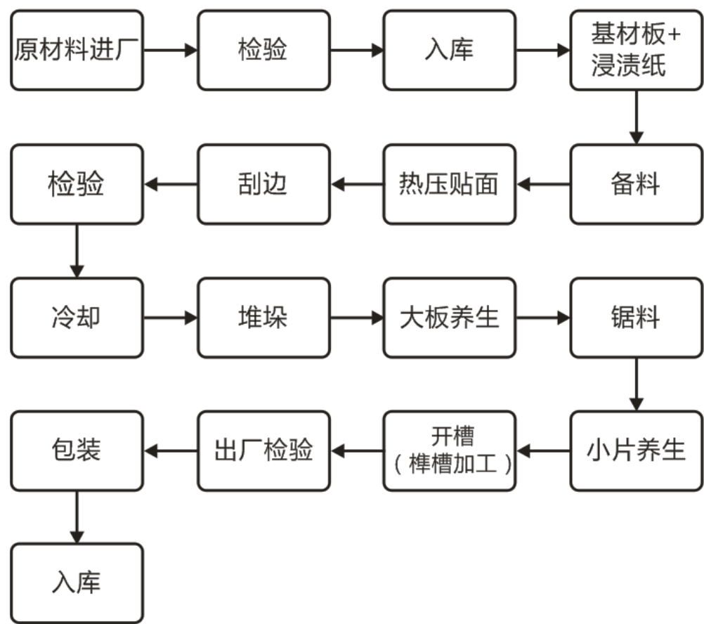
图 2 强化复合地板生产流程图
