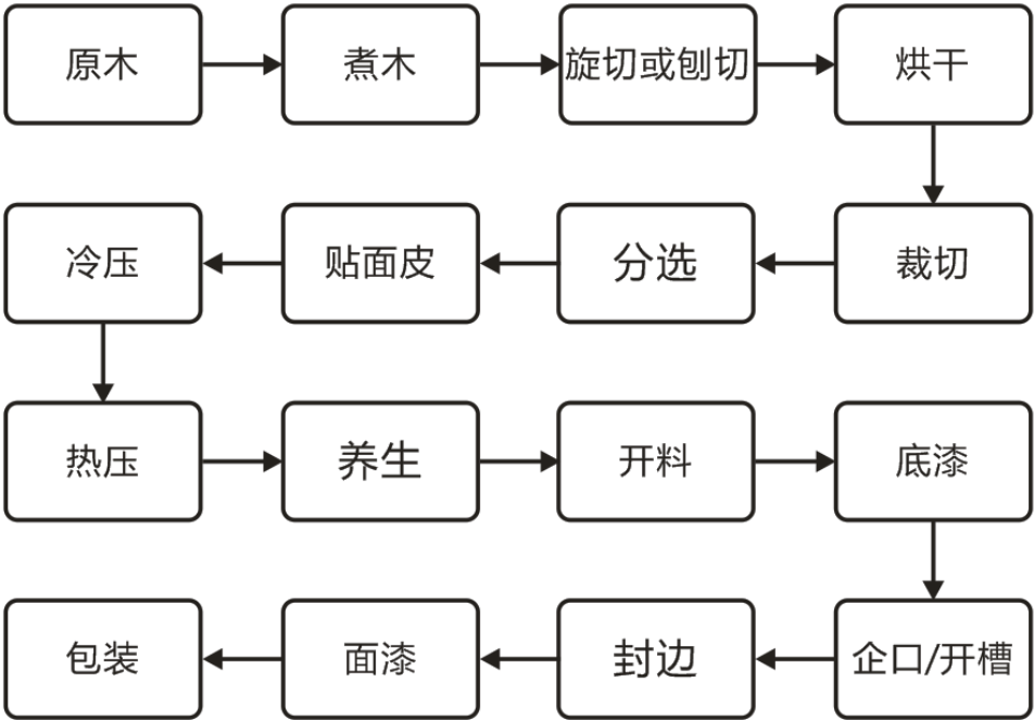
图 3 多层实木复合地板生产流程图
