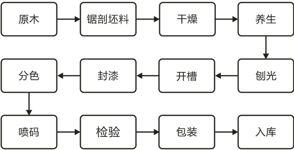
图 4 实木地板生产流程图
