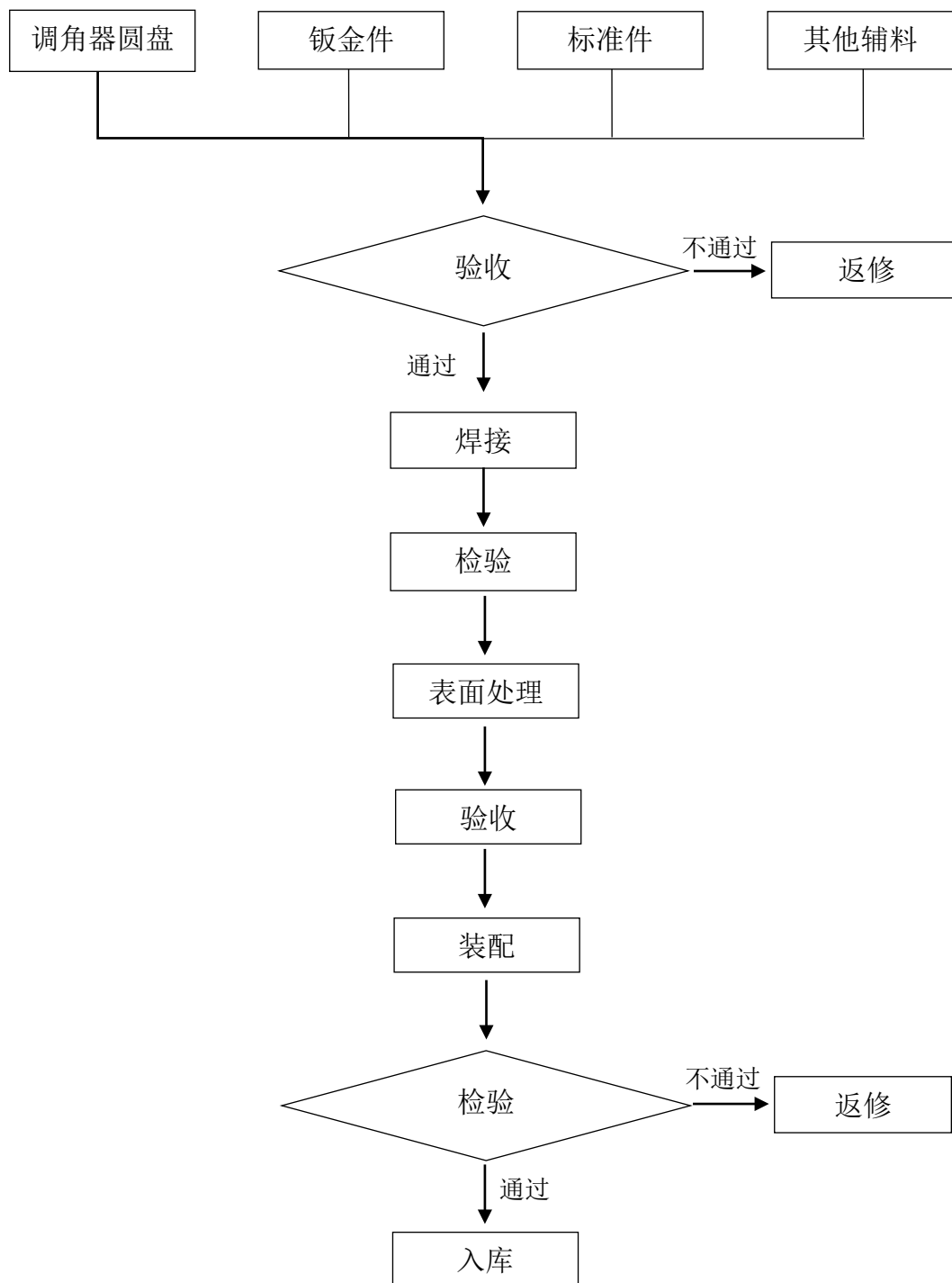
(3) 调角器生产流程图
