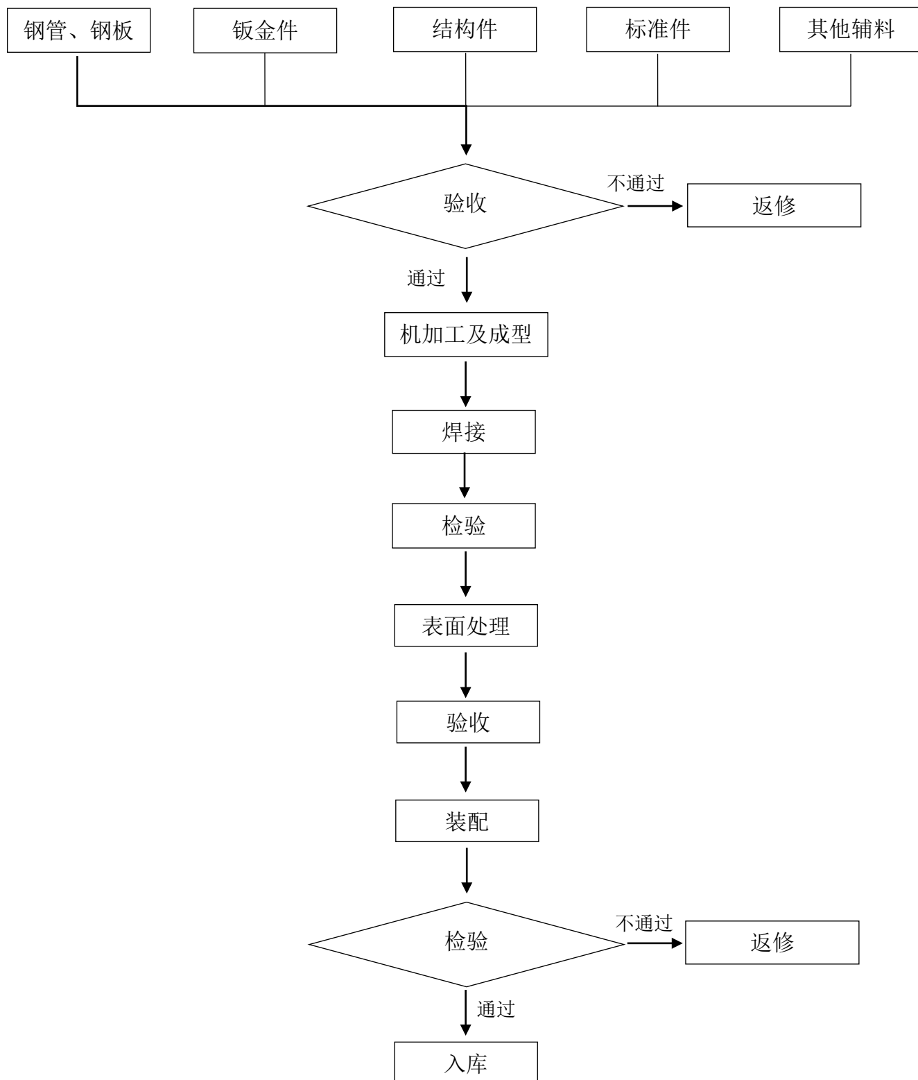
(2) 座椅骨架总成生产流程图
