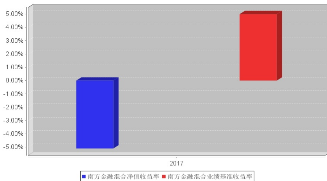
南方金融混合基金每年净值增长率与同期业绩比较基准收益率的对比图
