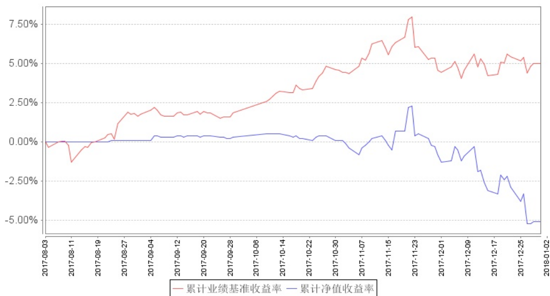
南方金融混合累计净值增长率与同期业绩比较基准收益率的历史走势对比图
