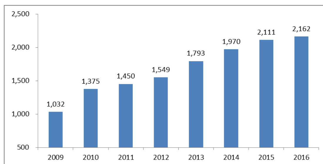
图：2009-2016 年我国乘用车销量（单位：万辆）
