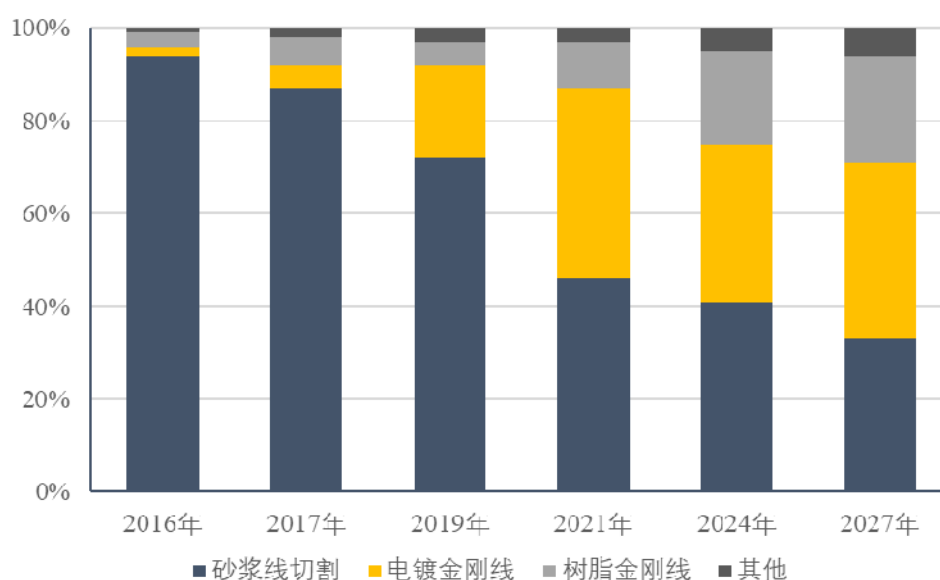
2016-2027 年不同硅片切割技术在多晶硅切片领域所占份额
