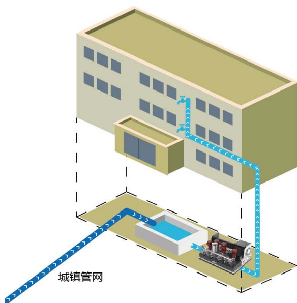
变频二次供水系统
