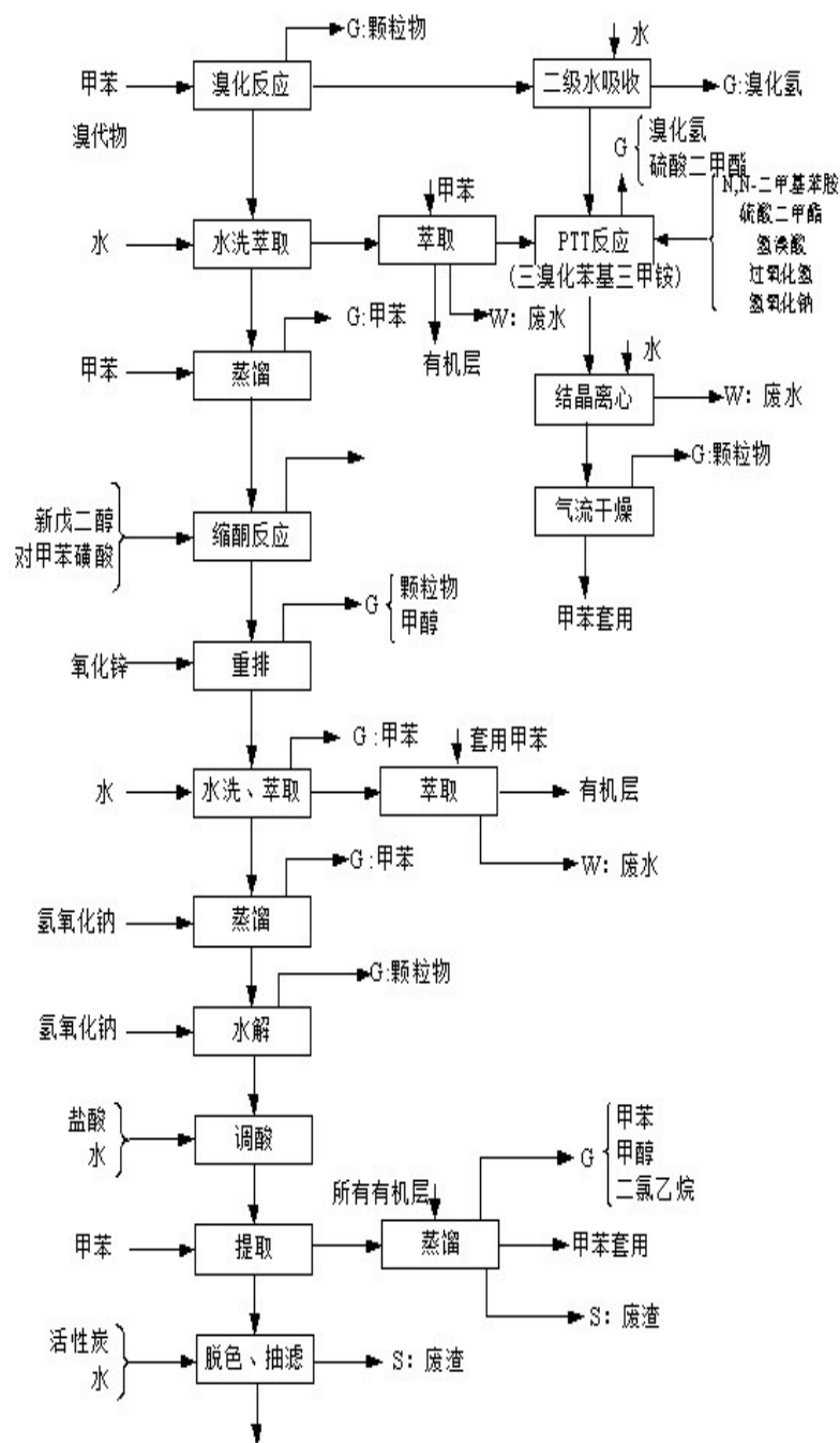
萘普生及其系列物工艺流程
