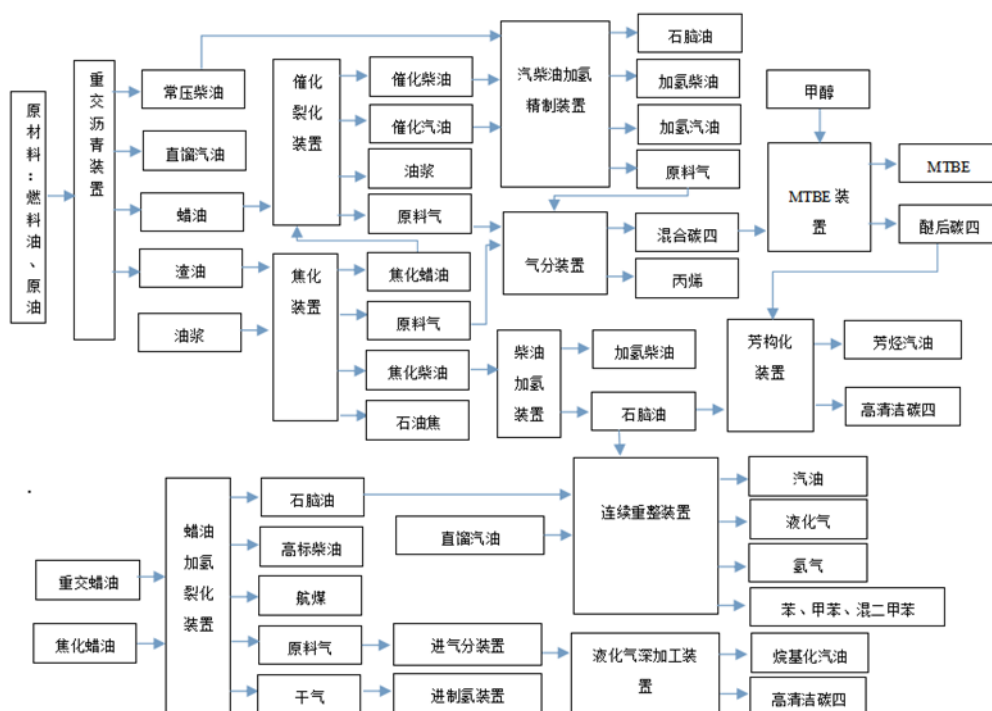
图：亚通石化主要装置工艺流程图
