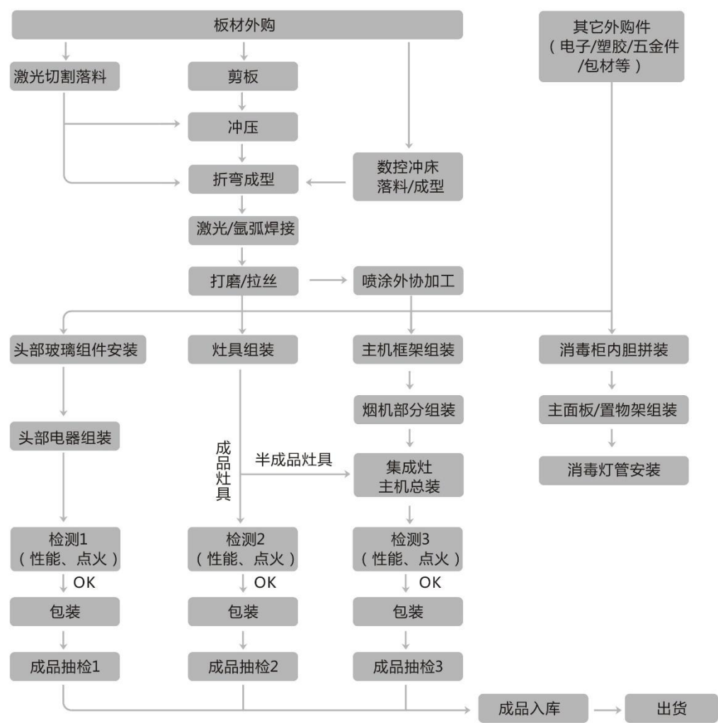
集成灶生产工艺流程图
