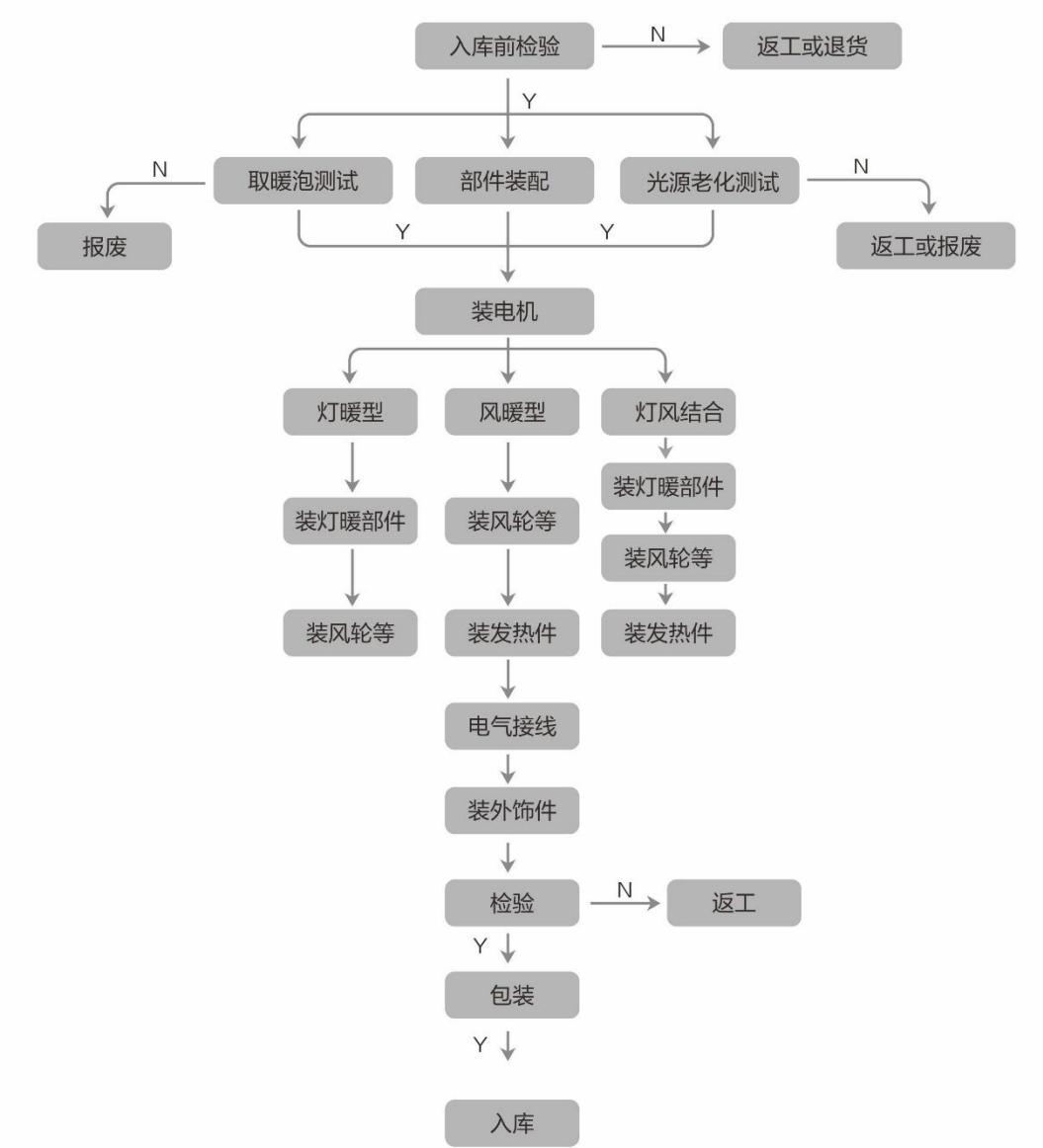
浴霸生产工艺流程图
