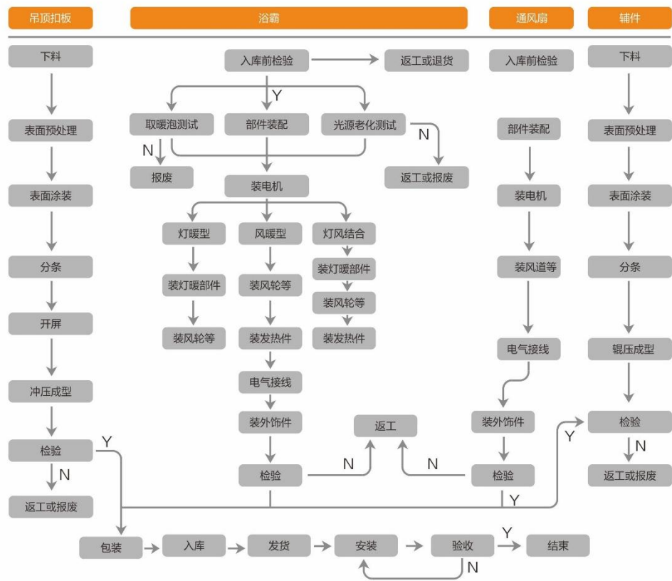
集成吊顶生产工艺流程图
