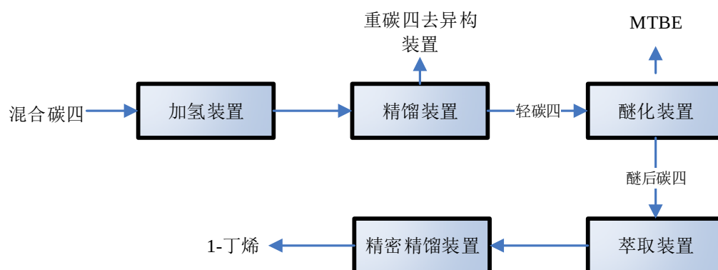
碳四加工工艺流程简图
