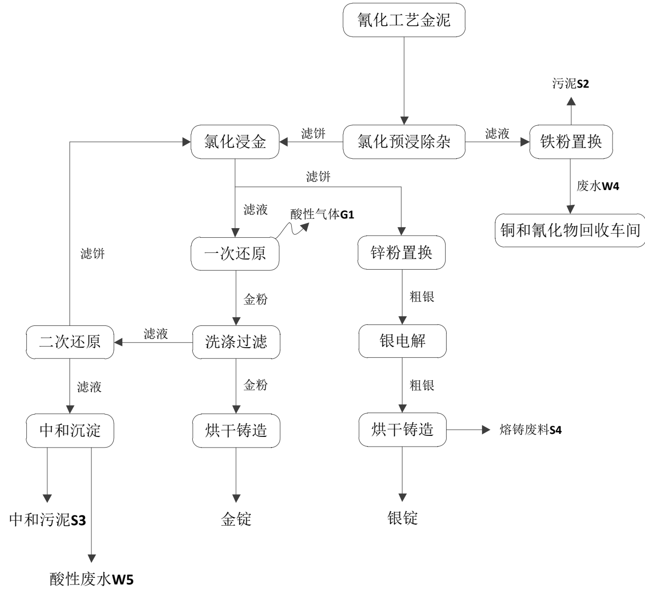
金泥精炼工艺流程图
