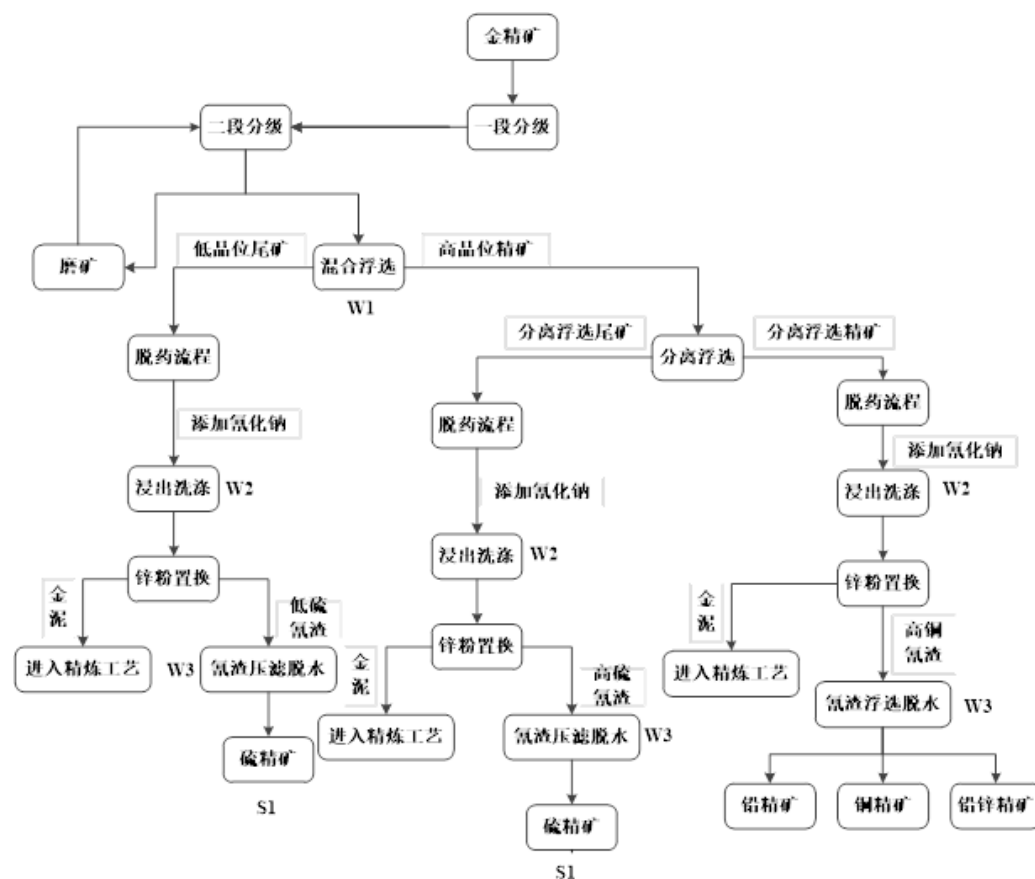
氰化工艺流程图
