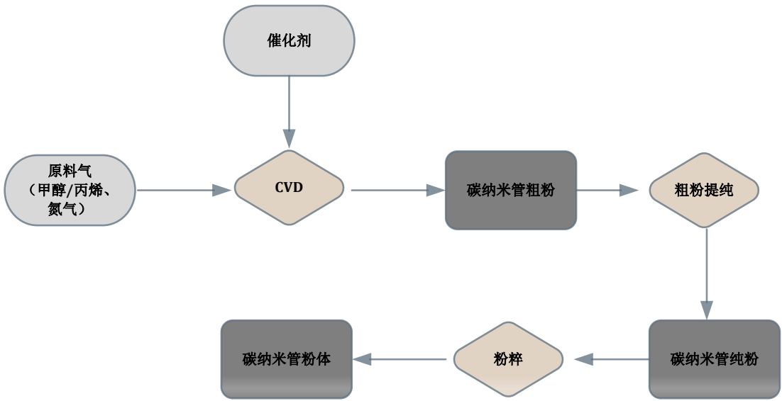
（1）年产 3,000 吨碳纳米管工艺流程图
