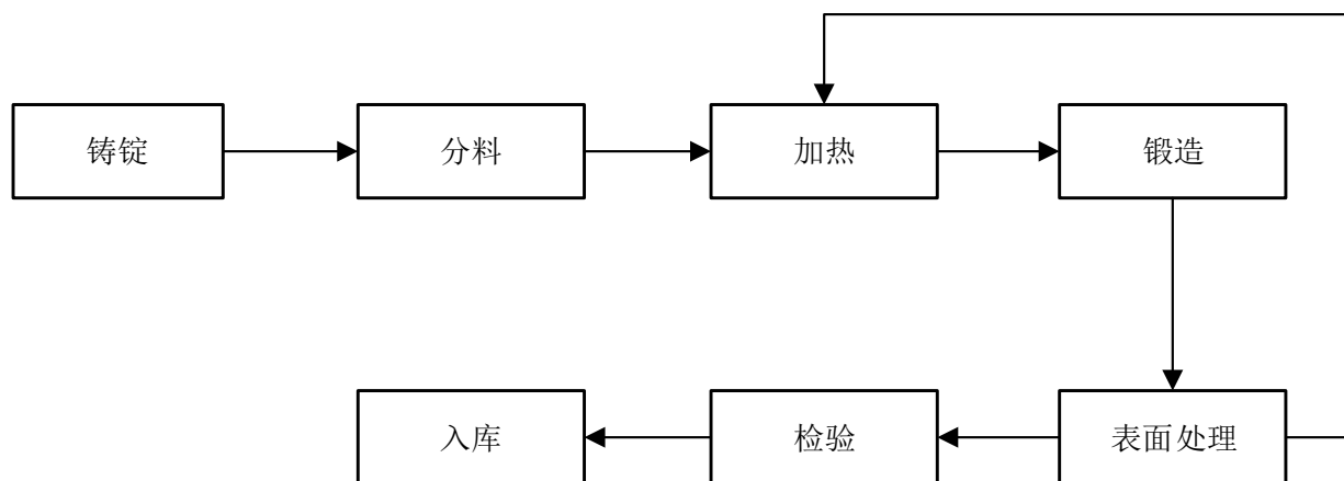
(2) 二厂（自由锻造厂）流程图
